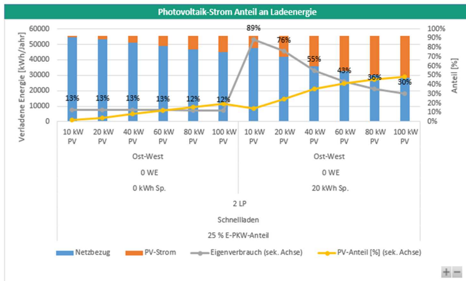
Abbildung 38: Eigenverbrauchsanteile ohne (links) und mit Batteriespeicher (rechts) am Standort Gehlsdorf.
