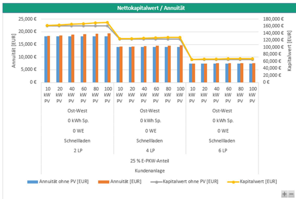
Abbildung 35: Wirtschaftlichkeit halböffentlicher Schnell-Ladeinfrastruktur am Standort Mittelmole, bei Netzstromkosten von 20 ct/kWh und PV-Investitionskosten von 1.400 €/kW.
