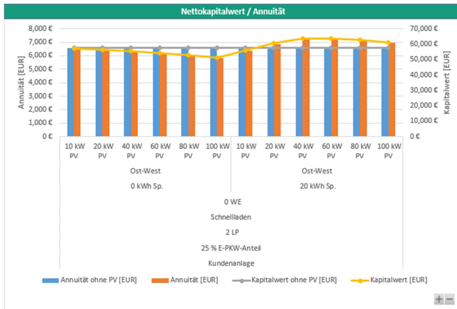
Abbildung 39: Wirtschaftlichkeit halböffentlicher Schnell-Ladeinfrastruktur am Standort Sporthalle Gehlsdorf, bei Netzstromkosten von 20 ct/kWh und PV-Investitionskosten von 1.400 €/kW, mit Berücksichtigung eines Batteriespeicher mit Investitionskosten von 700 €/kWh.
