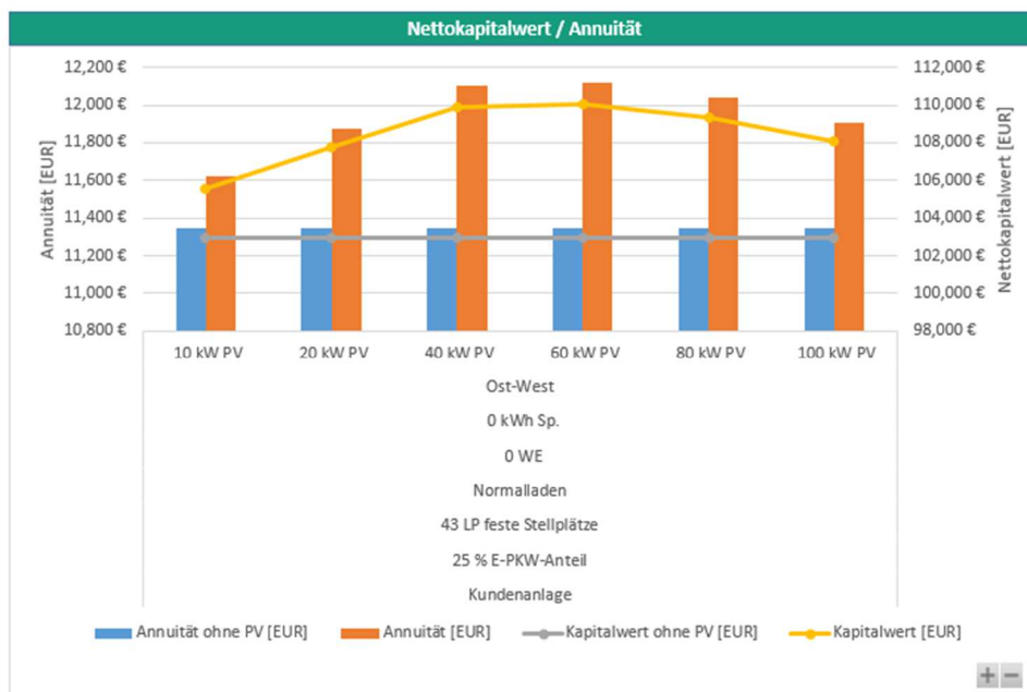
Abbildung 24: Vergleich des Nettokapitalwertes und der Annuität mit und ohne Photovoltaik-Integration.
