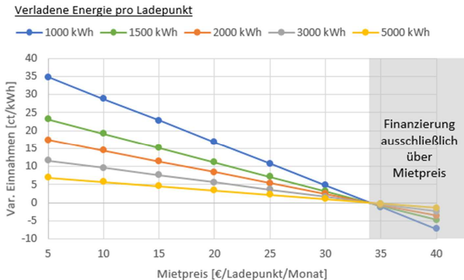
Abbildung 19: Refinanzierung der Investitionskosten einer privaten Ladeinfrastruktur (AC) über benutzungsabhängige Einnahmen, sowie einen monatlichen Mietpreis, in Abhängigkeit der Auslastung und unter der Annahme von 20 Ladepunkten und einem kalkulatorischen Zinssatz von 3 %.
