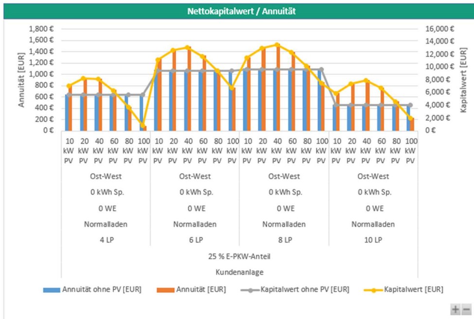
Abbildung 29: Vergleich der Wirtschaftlichkeit gemeinsam genutzter Ladepunkte mit normaler Ladegeschwindigkeit mit und ohne Photovoltaik-Anlage bei Investitionskosten von 1.400 €/kW und einem Netzstrompreis von 20 ct/kWh.
