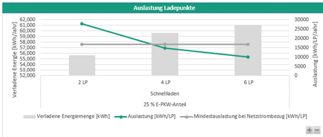
Abbildung 36: Auslastung für Ladeinfrastruktur mit schneller Ladegeschwindigkeit für unterschiedliche Anzahl an Ladepunkten am Standort Gehlsdorf.
