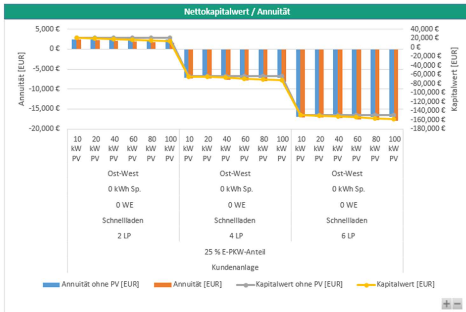
Abbildung 47: Wirtschaftlichkeit einer Schnelllade-Infrastruktur am Standort "Platz der Freundschaft" für alle Nachfragesegmente inkl. WIRO-Bewohner und Gewerbe.
