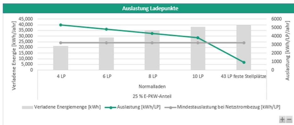
Abbildung 25: Auslastung der Normal-Ladeinfrastruktur für unterschiedliche Anzahl an Ladepunkten bei gemeinsamer und privater Nutzung (rechter Balken).
