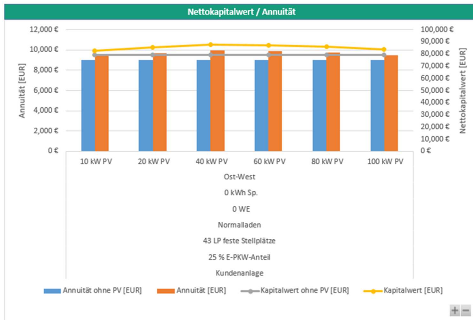
Abbildung 28: Vergleich der Wirtschaftlichkeit privater Ladepunkte mit und ohne Photovoltaik-Anlage bei Investitionskosten von 1.400 €/kW und einem Netzstrompreis von 25 ct/kWh und Ladepunkt-Miete.
