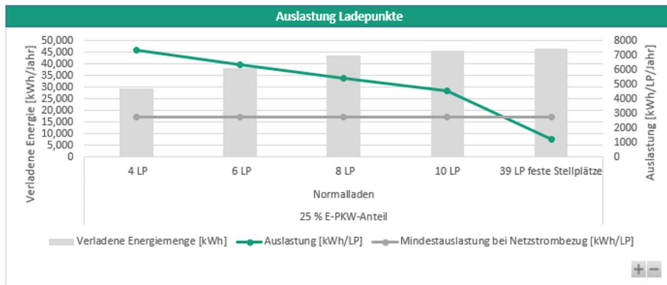
Abbildung 48: Auslastung einer Normallade-Infrastruktur am Standort "Platz der Freundschaft" für alle Nachfragesegmente inkl. WIRO-Bewohner und Gewerbe.
