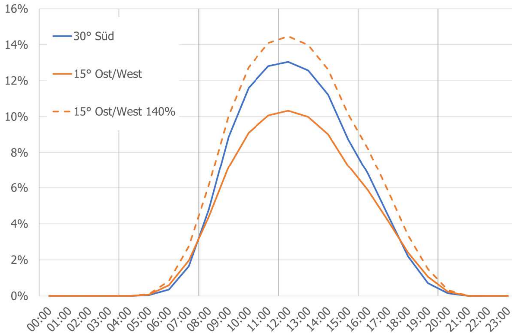
Abbildung 11: Tageszeitliche Verteilung des Stromertrags bei Photovoltaik in Abhängigkeit von der Ausrichtung der Paneele, Jahresmittel, unter Berücksichtigung der Sommerzeit
