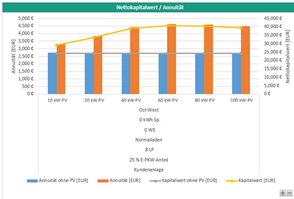
Abbildung 33: Vergleich der Wirtschaftlichkeit gemeinsam genutzter Normal-Ladepunkte, unter Einbeziehung weiterer Nachfragesegmente, mit und ohne Photovoltaik-Anlage bei Investitionskosten von 1.400 €/kW und einem Netzstrompreis von 25 ct/kWh.
