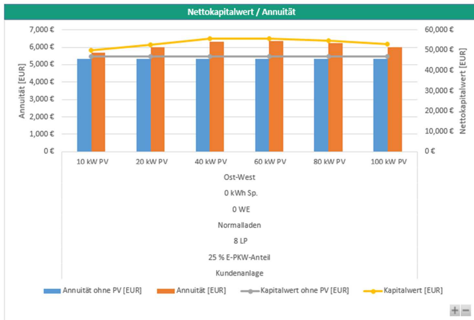
Abbildung 32: Vergleich der Wirtschaftlichkeit gemeinsam genutzter Normal-Ladepunkte, unter Einbeziehung weiterer Nachfragesegmente, mit und ohne Photovoltaik-Anlage bei Investitionskosten von 1.400 €/kW und einem Netzstrompreis von 20 ct/kWh.
