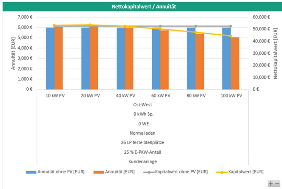
Abbildung 45: Vergleich der Wirtschaftlichkeit privater Ladepunkte mit und ohne Photovoltaik-Anlage bei Investitionskosten von 1.400 €/kW und einem Netzstrompreis von 25 ct/kWh und Ladepunkt-Miete.
