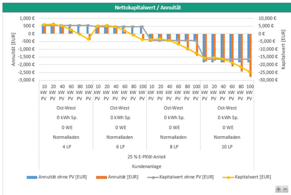
Abbildung 44: Wirtschaftlichkeit einer Normallade-Infrastruktur am Standort "Platz der Freundschaft" für die WIRO-Bewohner.
