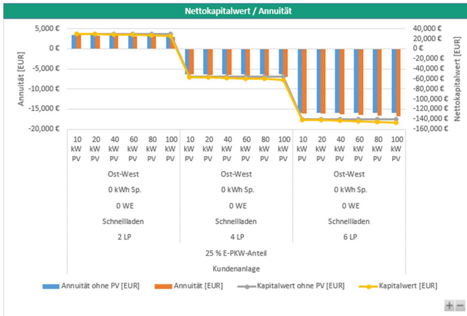
Abbildung 31: Vergleich der Wirtschaftlichkeit gemeinsam genutzter Ladepunkte, unter Einbeziehung weiterer Nachfragesegmente, mit hoher Ladegeschwindigkeit mit und ohne Photovoltaik-Anlage bei Investitionskosten von 1.400 €/kW und einem Netzstrompreis von 20 ct/kWh.
