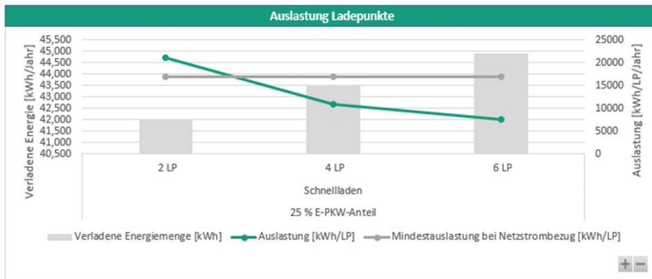
Abbildung 46: Auslastung einer Schnelllade-Infrastruktur am Standort "Platz der Freundschaft" für alle Nachfragesegmente inkl. WIRO-Bewohner und Gewerbe.
