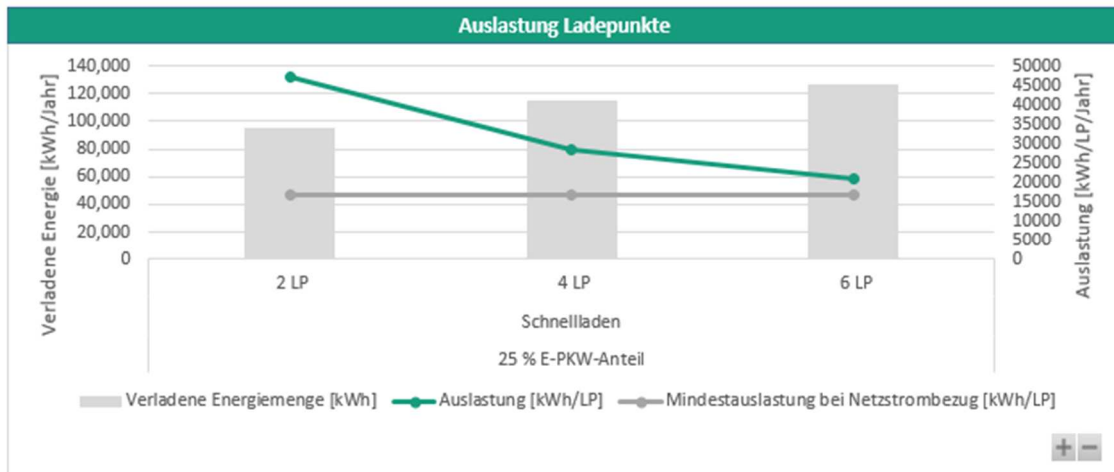
Abbildung 34: Auslastung für Ladeinfrastruktur mit schneller Ladegeschwindigkeit für unterschiedliche Anzahl an Ladepunkten am Standort Mittelmole.
