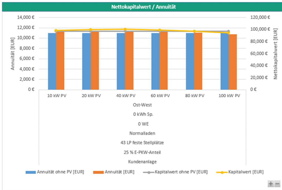
Abbildung 27: Vergleich der Wirtschaftlichkeit mit und ohne Photovoltaik-Anlage bei Investitionskosten von 1.400 €/kW und einem Netzstrompreis von 20 ct/kWh und Ladepunkt-Miete.
