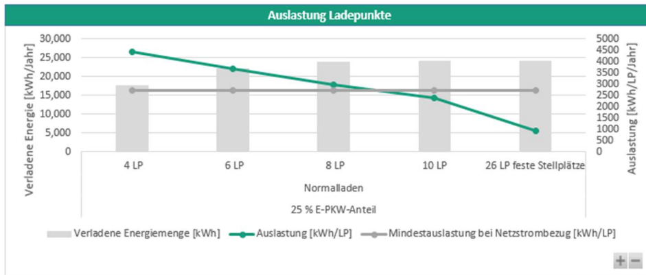
Abbildung 43: Auslastung einer Normallade-Infrastruktur am Standort "Platz der Freundschaft" für die WIRO-Bewohner.
