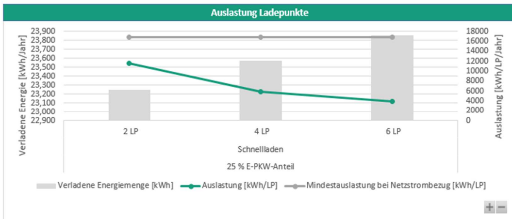
Abbildung 41: Auslastung einer Schnelllade-Infrastruktur am Standort "Platz der Freundschaft" für die WIRO-Bewohner.
