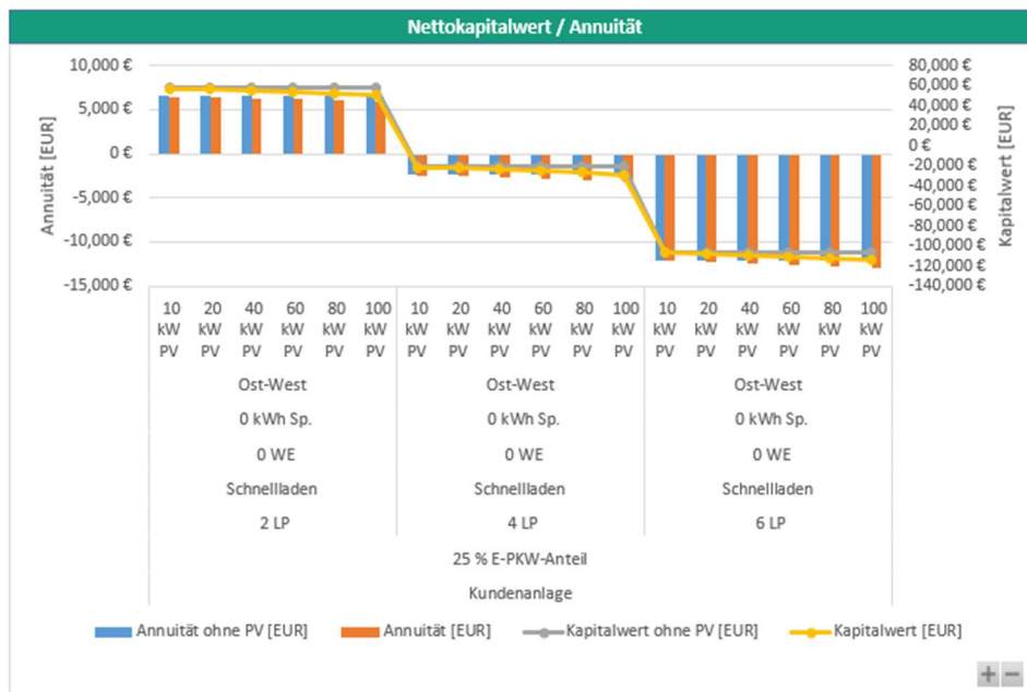
Abbildung 37: Wirtschaftlichkeit halböffentlicher Schnell-Ladeinfrastruktur am Standort Sporthalle Gehlsdorf, bei Netzstromkosten von 20 ct/kWh und PV-Investitionskosten von 1.400 €/kW.
