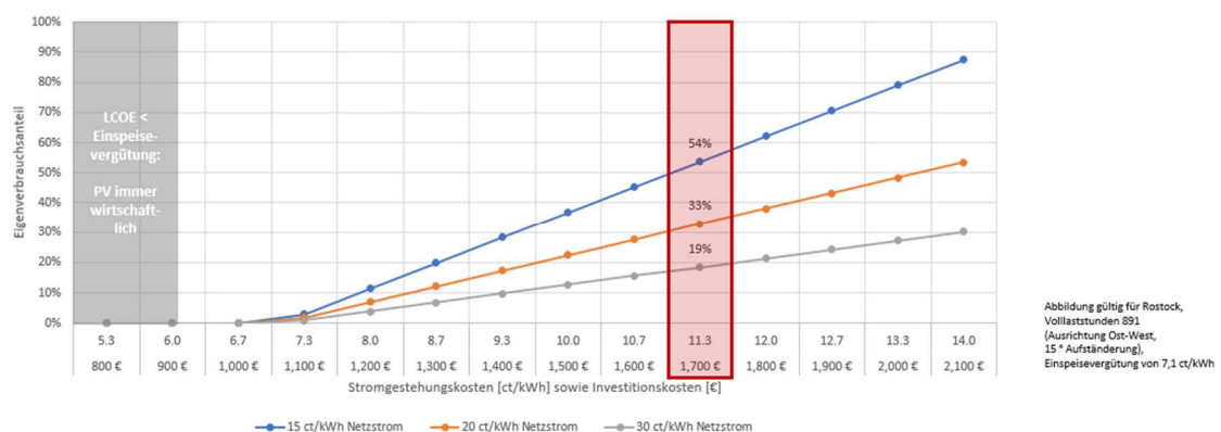
Abbildung 23: Stromgestehungskosten (LCOE) bei unterschiedlicher Höhe der Investitionskosten und notwendiger Eigenverbrauch in Abhängigkeit der Netzstromkosten.
