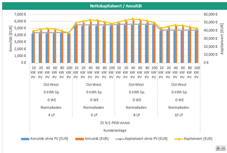
Abbildung 49: Wirtschaftlichkeit einer Normallade-Infrastruktur am Standort "Platz der Freundschaft" für alle Nachfragesegmente inkl. WIRO-Bewohner und Gewerbe.
