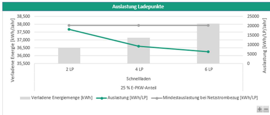
Abbildung 26: Auslastung der Schnell-Ladeinfrastruktur bei gemeinsamer Nutzung für unterschiedliche Anzahl an Ladepunkten.
